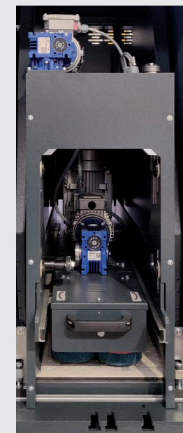
Gruppo spazzole tangenziali Tangential brushes unit Bürstenwalze tangential
